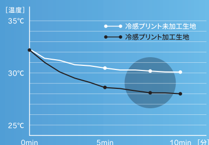
第三者機関による冷感プリントの吸水冷感試験グラフ (1分ごとの温度経過)
